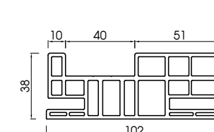
Đổ cửa 100H - PWF100H Door frame 100H - PWF100H
