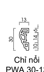
Chỉ nôi PWA 30-13 Decorative trim PWA 30-13
