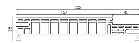
Đổ cửa 200 - PWF200 Door frame 200 - PWF200
