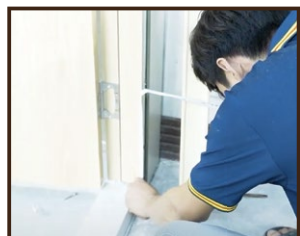
Bước 10: Đo cắt nẹp viền và gắn nẹp vào khung bao Step 10: Measure and cut the trims, then install them to the frame.
