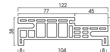
Đổ cửa 120 - PWF120 Door frame 120 - PWF120
