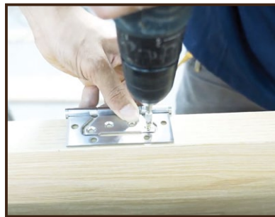
Bước 5: Bắn 3 bản lề vào cánh cửa theo đúng khoảng cách quy định Step 5: Install the 4 hinges to the door panel with the distance shown in the drawing.
