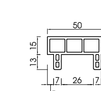
U đổ cửa 100H - PW 050 Door frame cap 100H - PW 050
