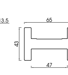
Thanh ray PABT 6543 Sliding door rail PABT 6543
