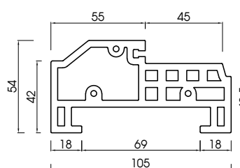
Đổ cửa 105 - PAK105 Door frame 105 - PAK105
