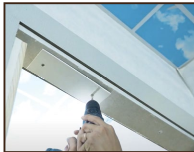
Bước 8: Lắp cây khung bao ngang Step 8: Install the horizontal frame.
