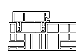
Bộ đổ cửa 100H Door frame set 100H
