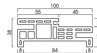
Đổ cửa 100 - PWF100 Door frame 100 - PWF100
