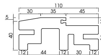
Đổ cửa 110 - PATB110 Door frame 110 - PATB110
